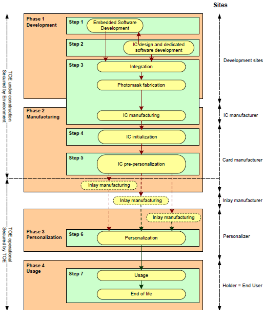
Figure 2 - Cycle de vie : Initialisation du module sur le site de GEMALTO
