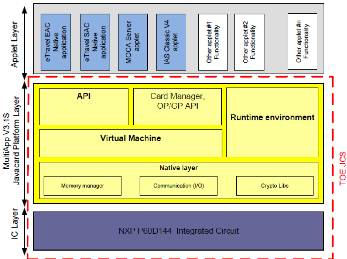
Figure 1 - Architecture et périmètre de la TOE
