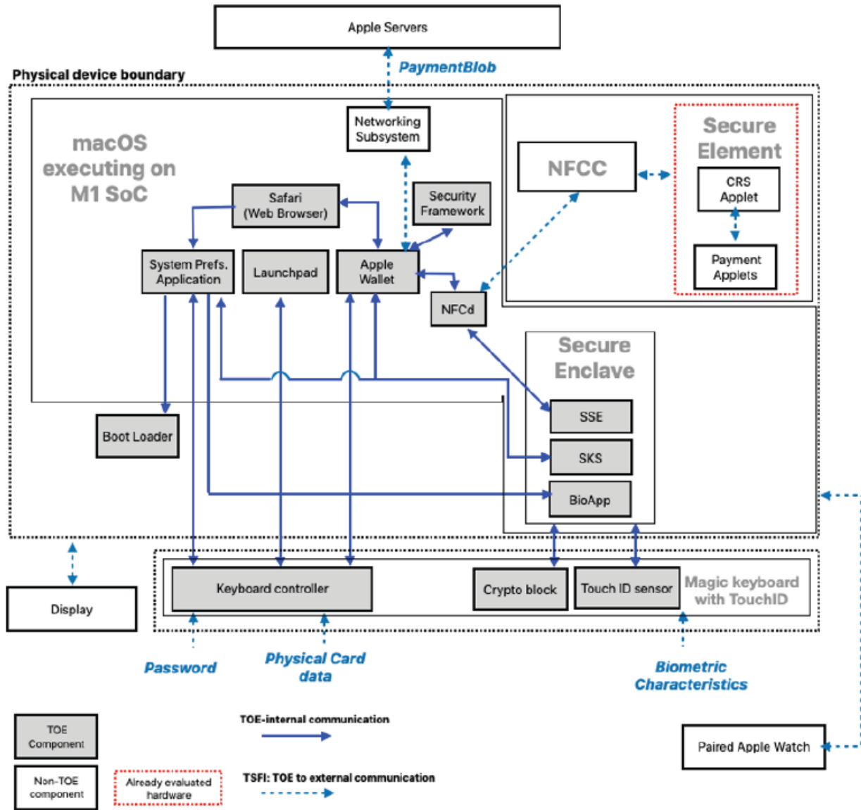
Figure 1 : Architecture du produit
